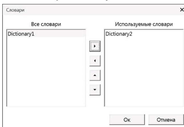
Рис. 4.29. Словари
