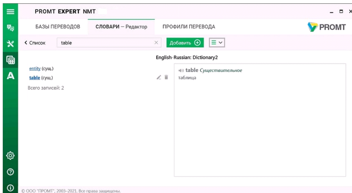
Рис. 4.26. Словари —Редактор
