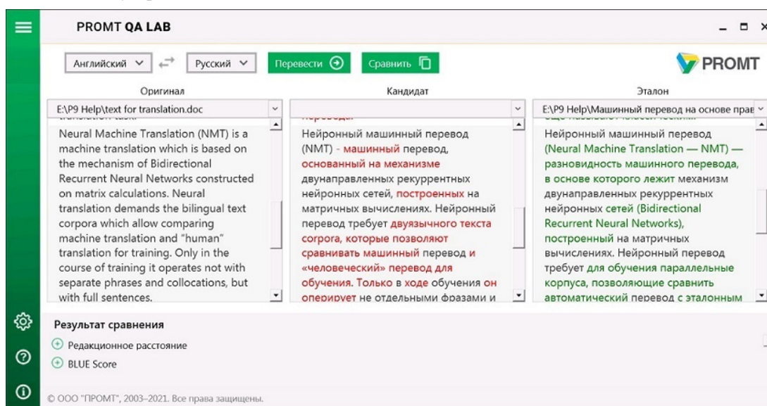
Рис. 6.3. Сравнение переводов
