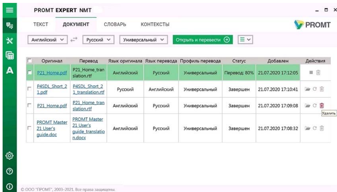
Рис. 4.11. Перевод документов
