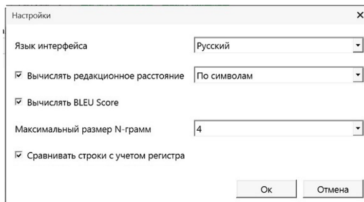
Рис. 6.4. Настройка приложения
