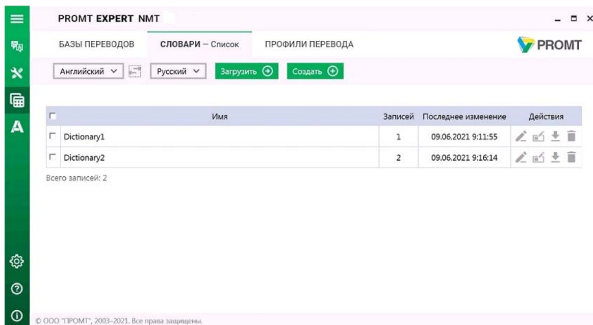
Рис. 4.25. Словари —Список
