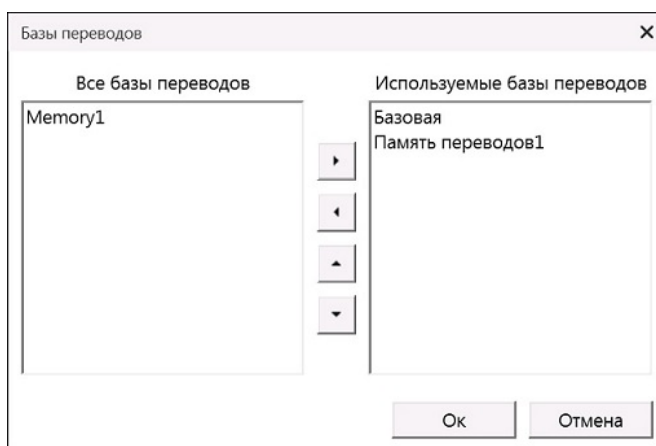
Рис. 4.30. Базы переводов
