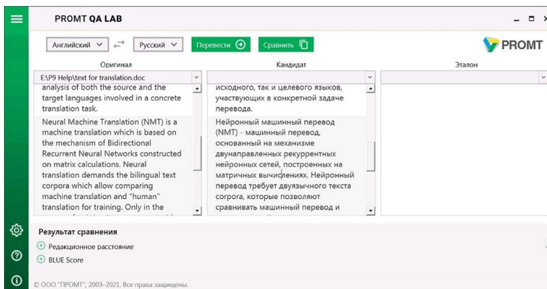
Рис. 6.2. Перевод текста
