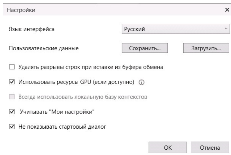
Рис. 4.36. Настройка приложения
